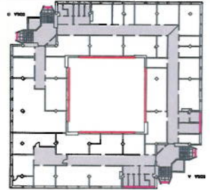
PIANO TERZO
